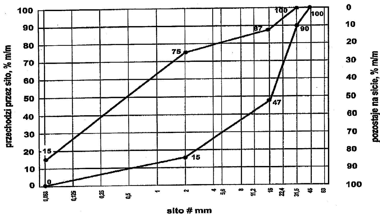
Rys. 2.7. Uziarnienie mieszanki niezwiązanej 0/31,5 do nawierzchni
