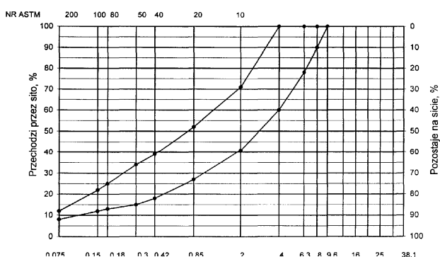
Rys. 3 Krzywe graniczne uziarnienia mieszanki mineralnej BA od 0 do 8mm, od 0 do 6,3 mm do warstwy ścieralnej nawierzchni drogi o obciążeniu ruchem dla KR1 lub KR2
