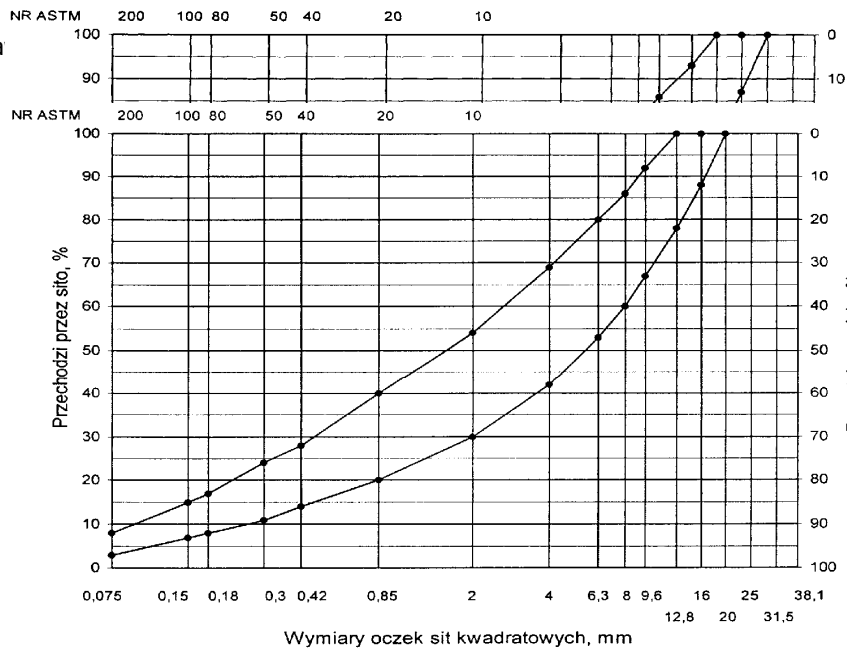
Rys. 9. Krzywe graniczne uziarnienia mieszanki mineralnej BA od 0 do 16 mm do warstwy wiążącej, wyrównawczej i wzmocniającej nawierzchni drogi o obciążeniu ruchem KR1 lub KR2
